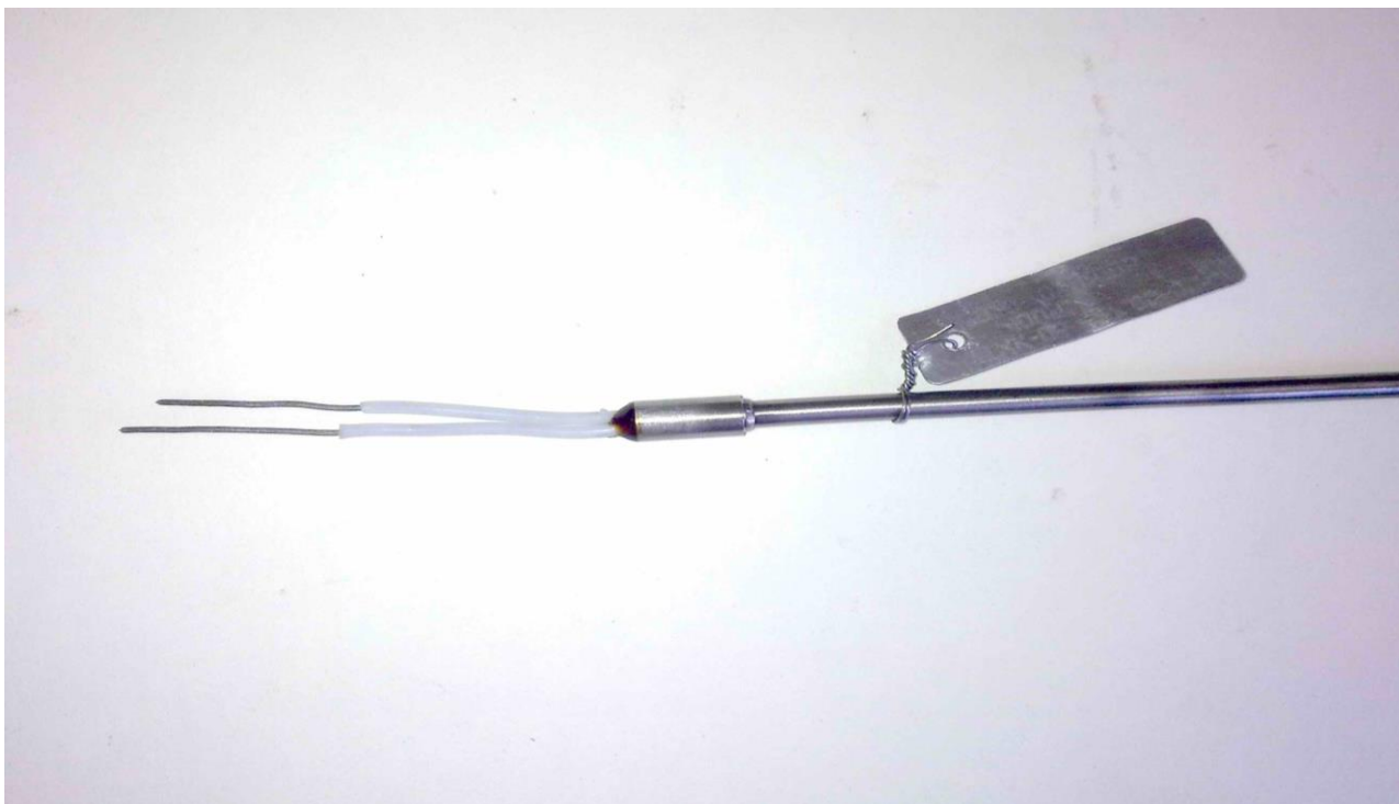
Рисунок 1 – ТП ТХК-05
