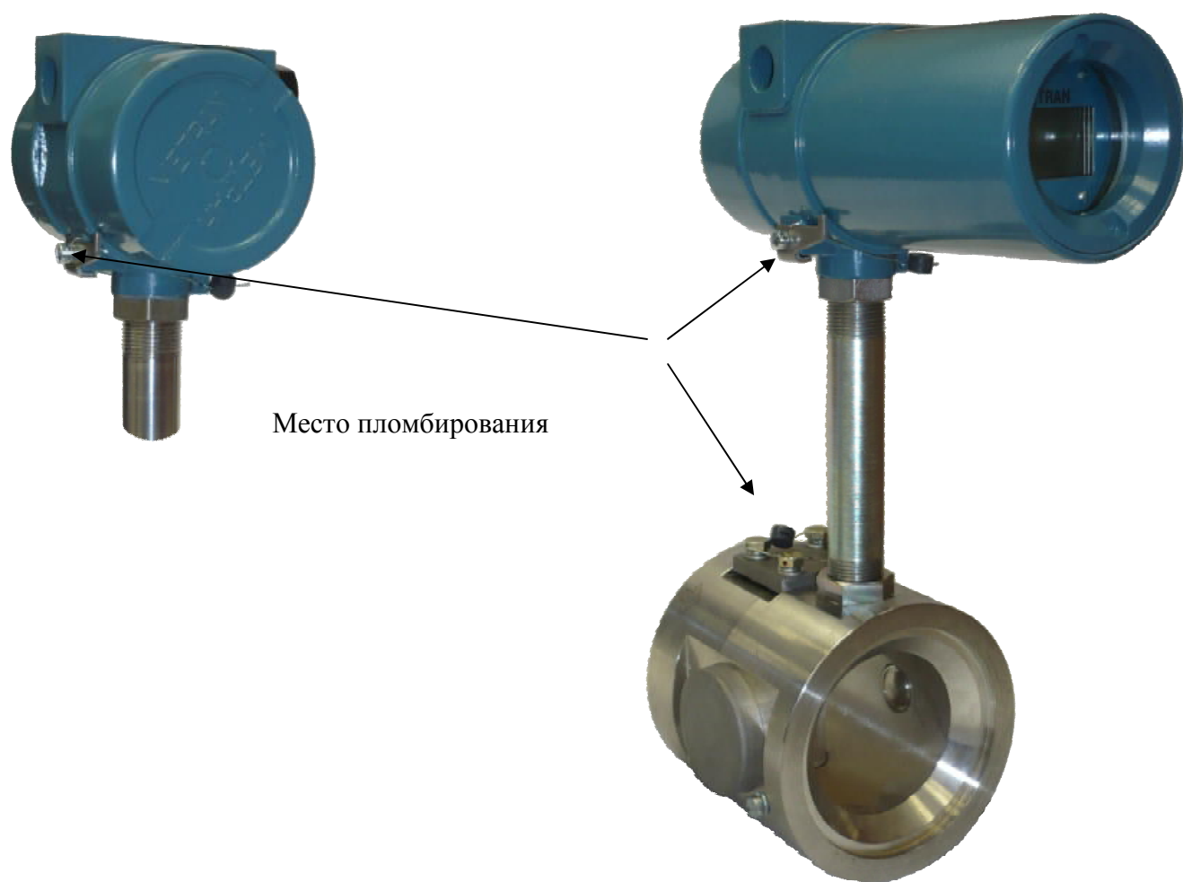
Рисунок 1 – Общий вид преобразователя с местами пломбирования
