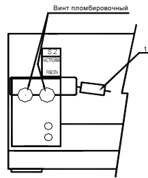
Рисунок 2.5 Схема пломбирования микропроцессора отсчетного устройства «Топаз»
