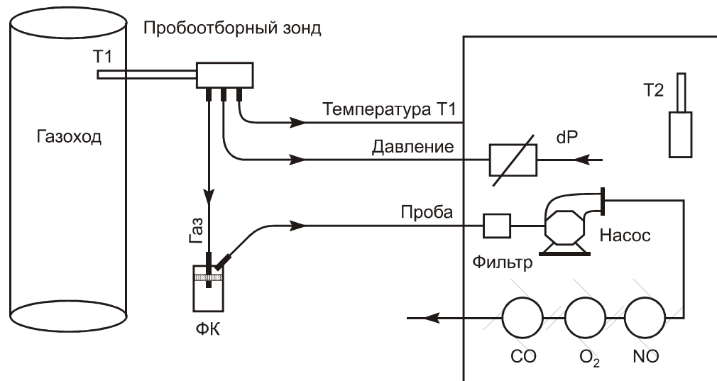
Рис. 1. Схема газового модуля газоанализатора «Топогаз-01».
