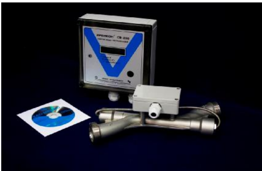
Рисунок 1 – Внешний вид счетчика Ду32 осевого типа одноканального
