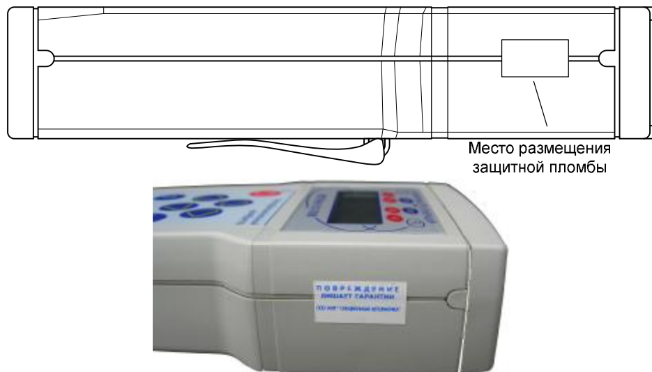
Рисунок 2 – Схема и внешний вид пломбировки калибратора от несанкционированного доступа.
