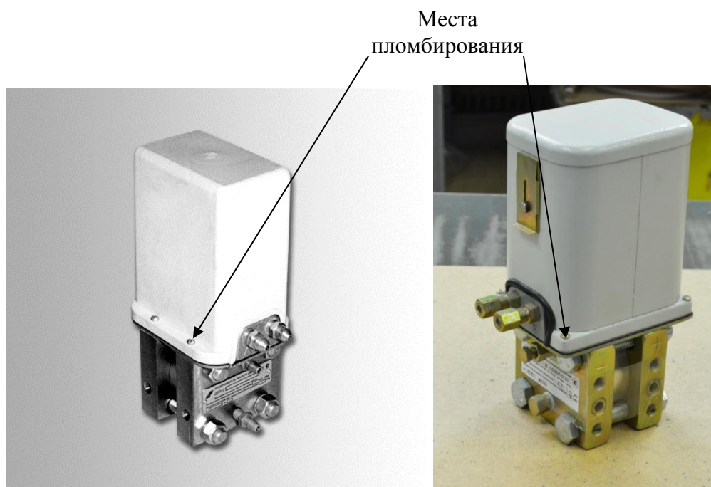
Рисунок 1 - Внешний вид преобразователя пневматического разности давлений ДПП-2М в пластиковом и металлическом кожухах
