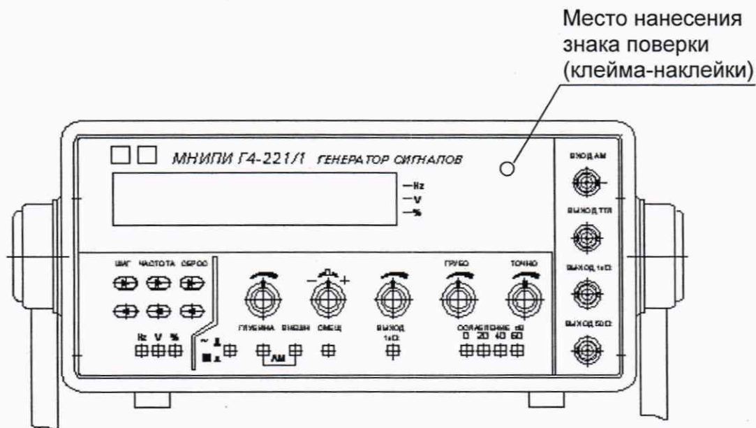
Рисунок А.1 - Передняя панель генераторов сигналов Г4-221 и Г4-221/1
