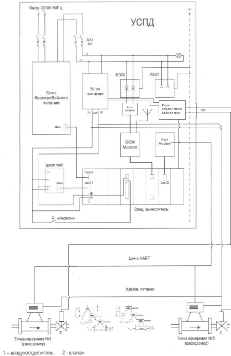
Комплекс измерительный автоматизированного учета алкоголя "БАКУС-2006" (Схема структурная)
