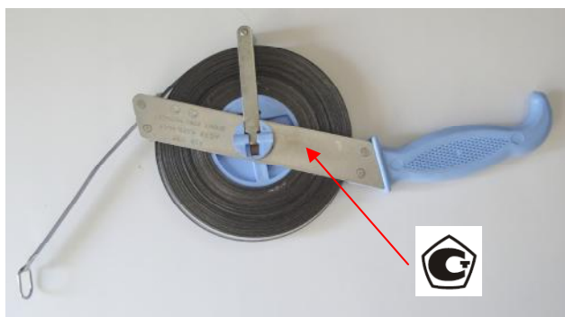
Рисунок 1 – Рулетки измерительные металлические Р30УЗК
