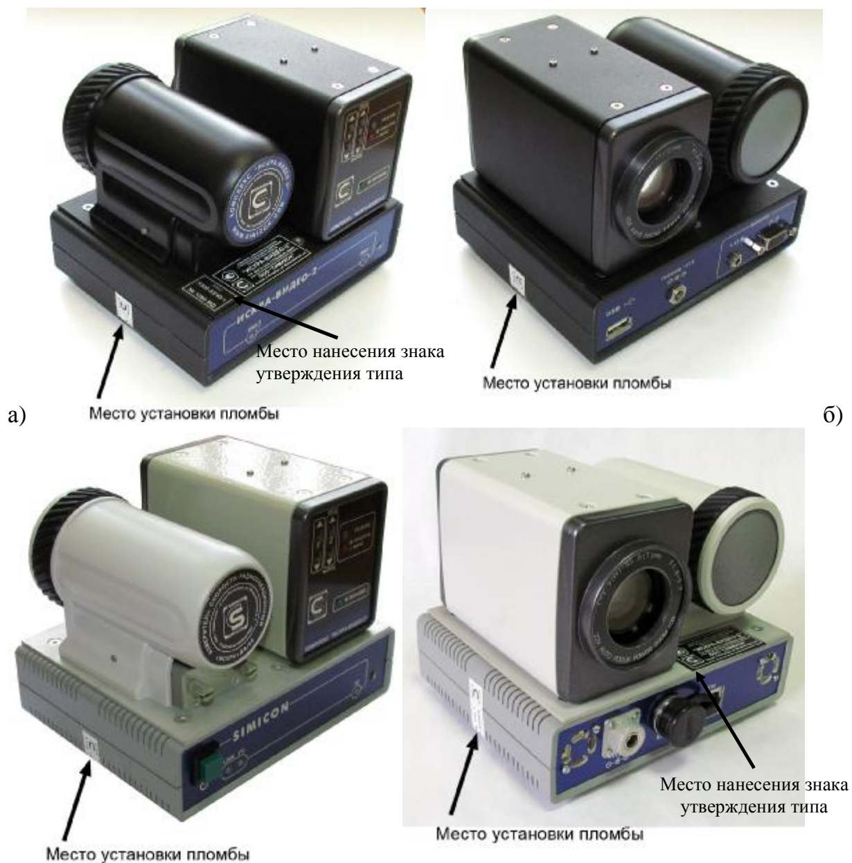
Рисунок 1 – Общий вид комплекса измерения скорости и регистрации видеоизображения транспортных средств «Искра-видео-2»: а) исполнение «МД»; б) исполнение «КД».
