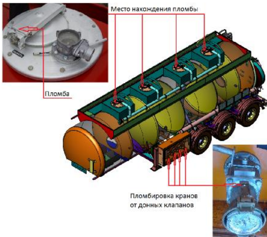
Рисунок 2 - Места пломбирования полуприцепов-цистерн
