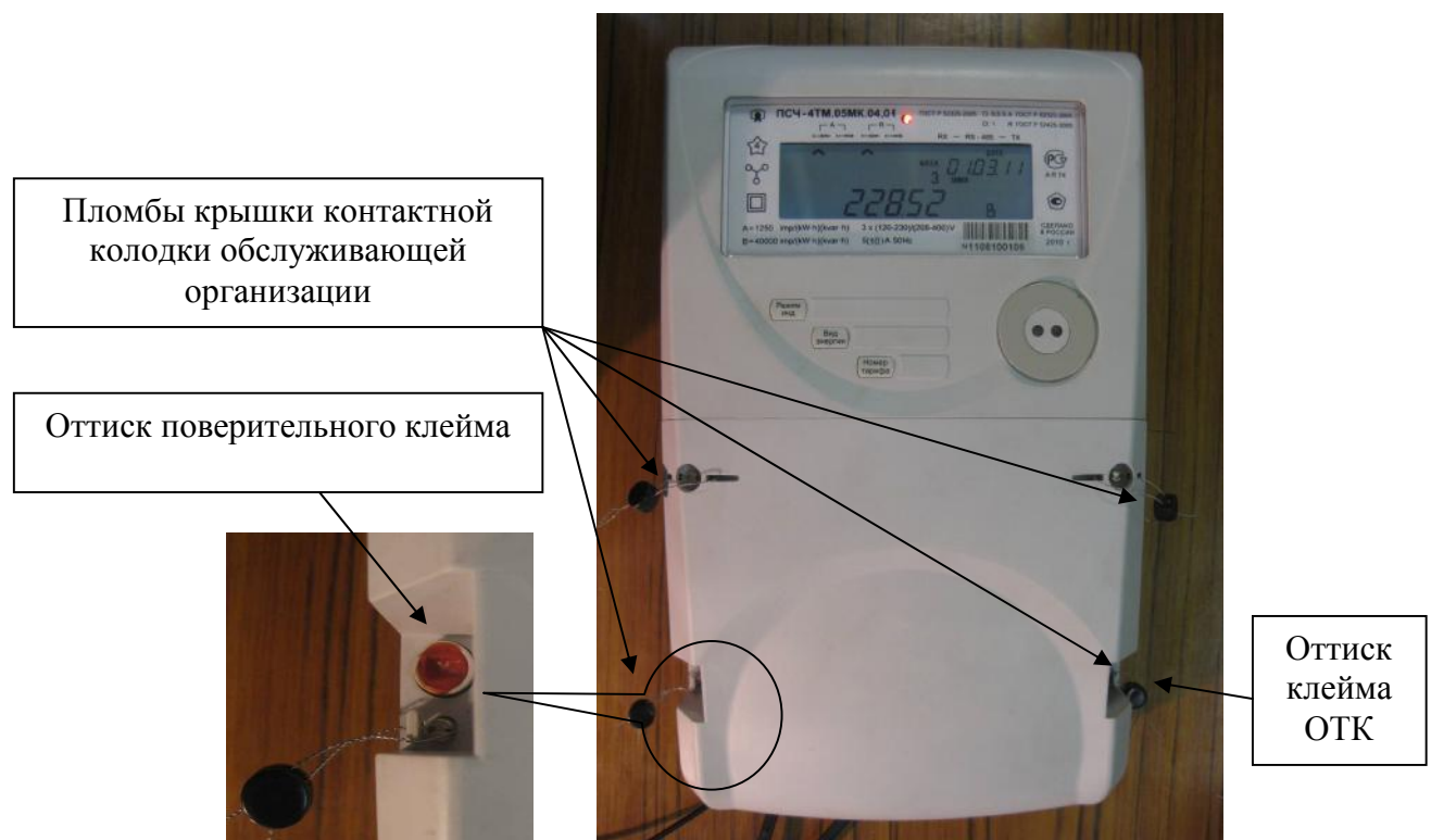
Рисунок 1 – Внешний вид счетчика с закрытой крышкой контактной колодки и схема пломбирования
