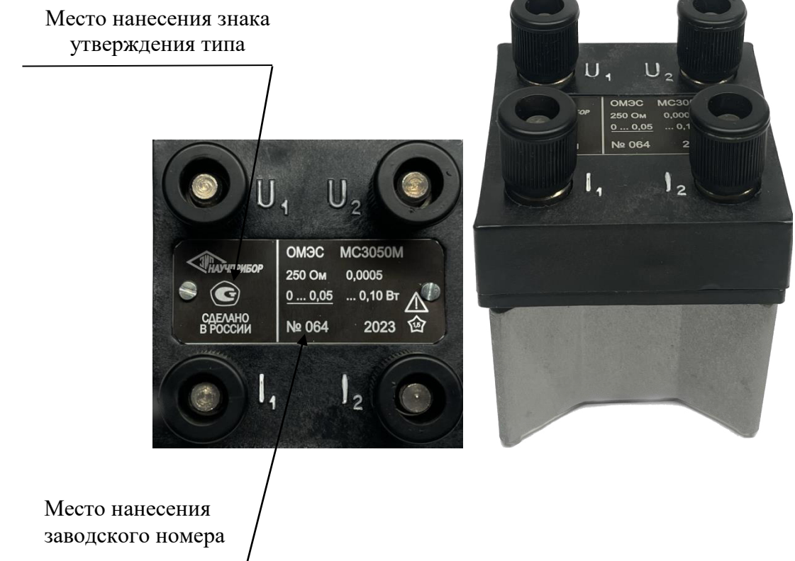
Рисунок 1 - Общий вид МС3050М-1
