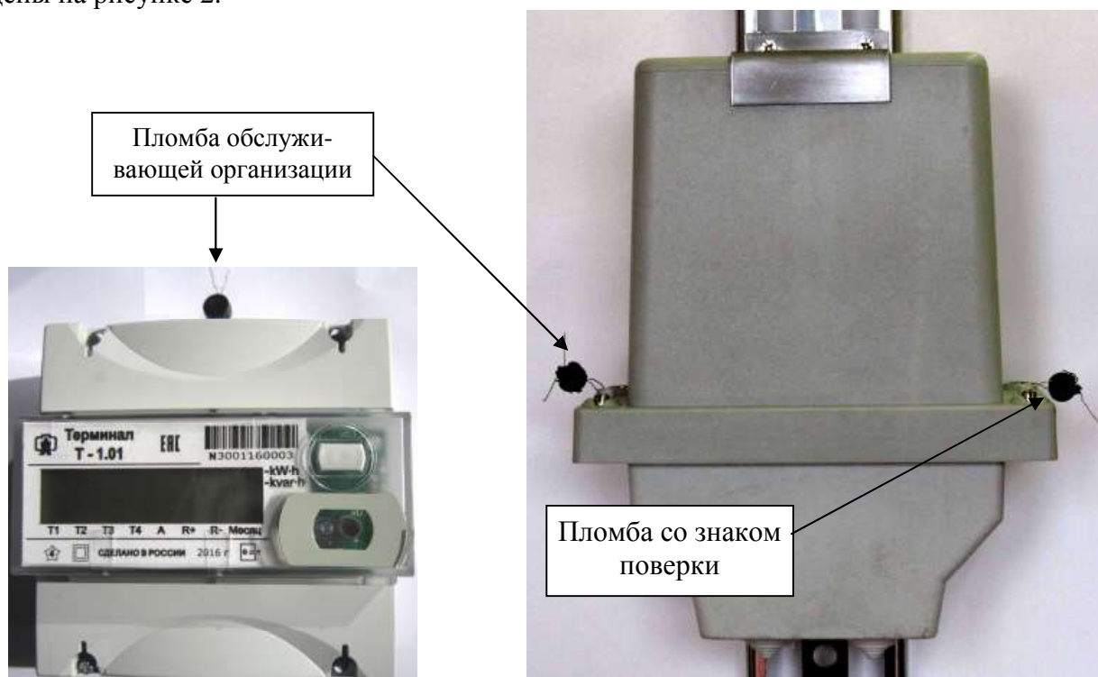
Рисунок 2 - Внешний вид счетчиков наружной установки и схема пломбирования
