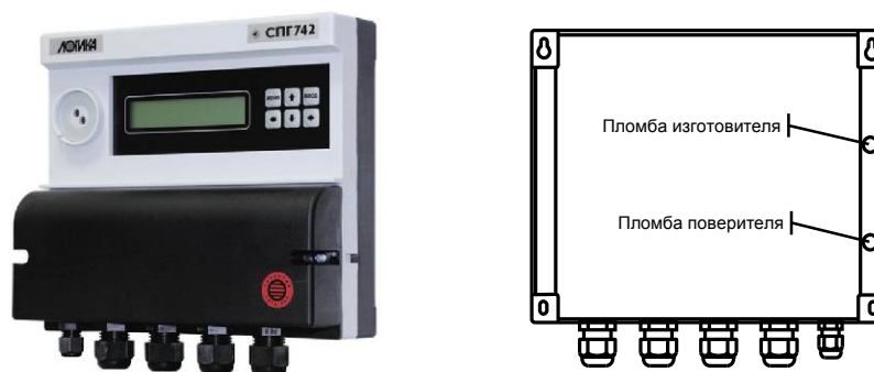
Рисунок 1 - Общий вид и схема пломбирования (вид сзади)
