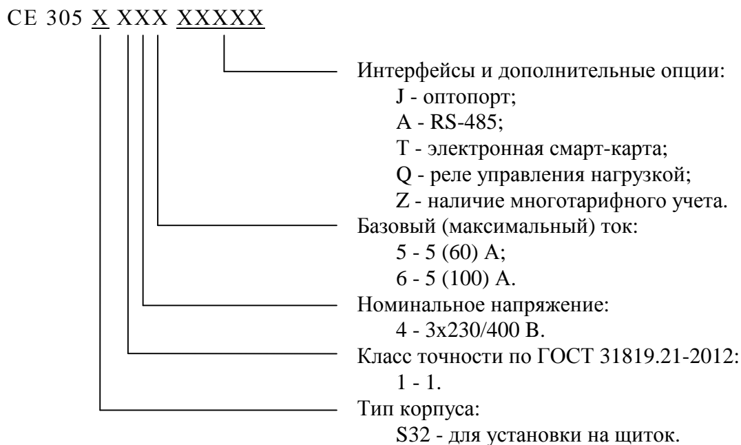
Рисунок 1 - Структура условного обозначения счётчика
