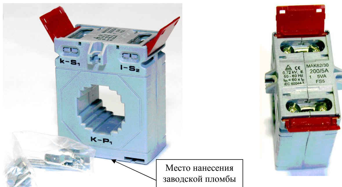
Рисунок 2 - Общий вид трансформаторов и схема пломбировки
