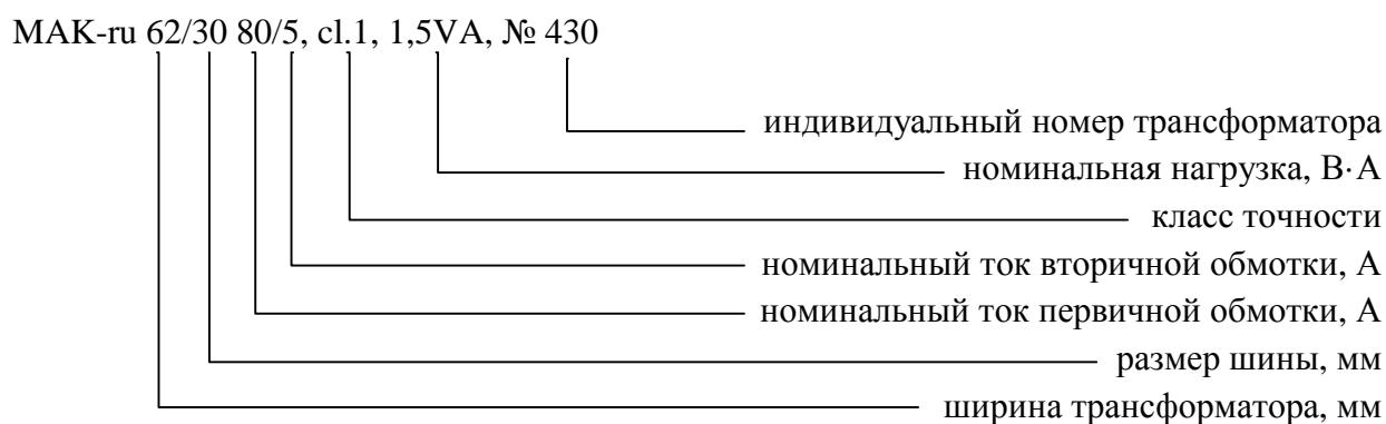
Рисунок 1 - Структура обозначения трансформаторов
