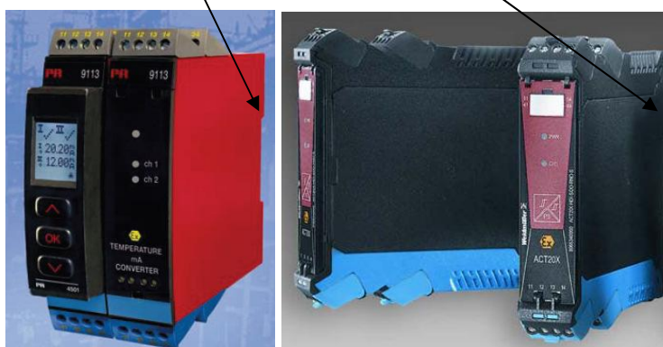
Рис.4 Внешний вид преобразователей измерительных PR серии 9.
