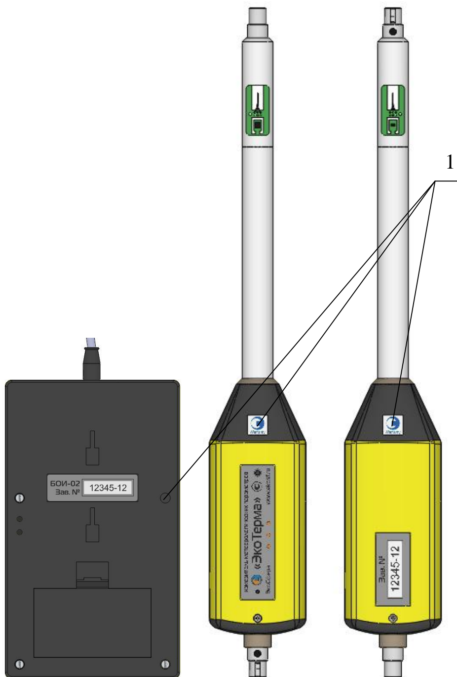
Рисунок 3. Схема пломбирования станций «ЭкоТерма-02» (измерительный блок показан спереди и сзади) Пломбы – 1
