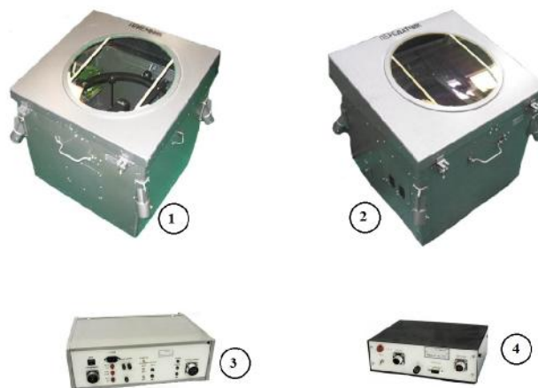
Рис. 1 Датчики высоты облаков ДВО-2 1 – приемник, 2 – излучатель, 3 – блок измерительный, 4 – пульт дистанционный
