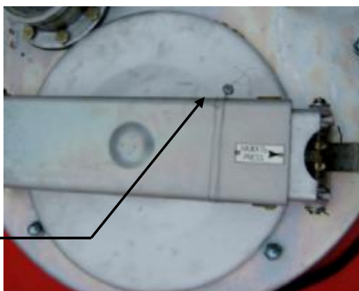
Рисунок 4 – Запорный механизм крышки заливной горловины ППЦ
