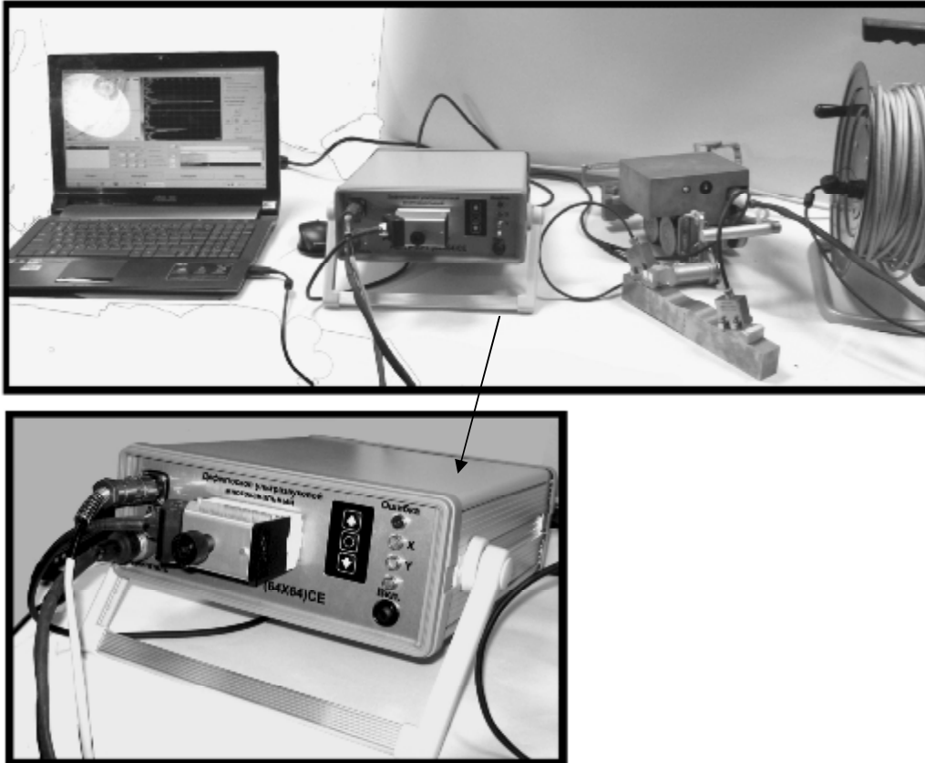
Рисунок 1 – Внешний вид управляющего компьютера, дефектоскопа, соединительных кабелей, СКУАР и АР на призмах
