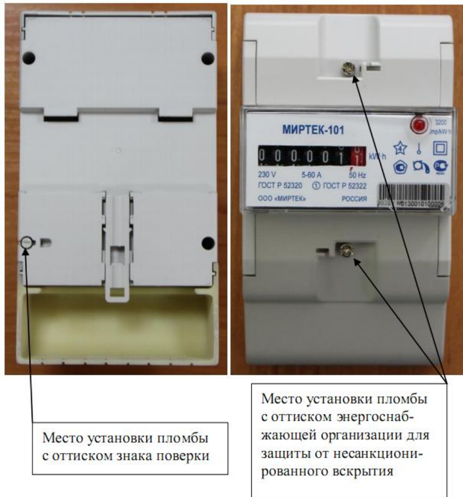
Рисунок 6 – Общий вид счетчика в корпусе модификации D4
