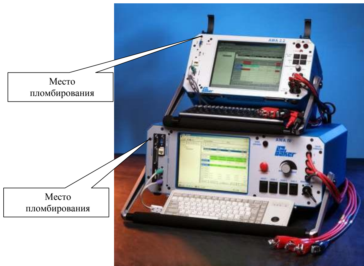
Рис. 1 – Внешний вид анализаторов
