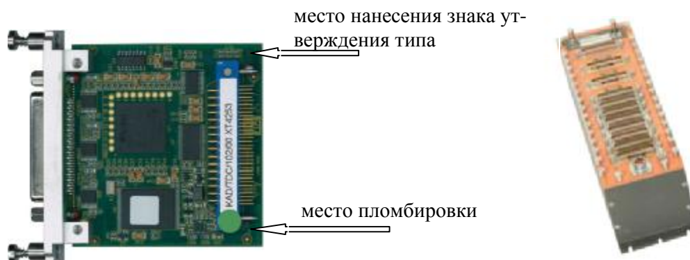
Рисунок 1 - Внешний вид модуля KAD/TDC/102/B и модуля KAD/TDC/102/B, установленного в блок базовый KAM/CHS/13U
