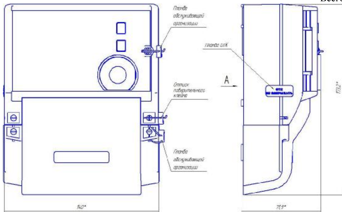
Рисунок 2 – Схема пломбирования счётчика
