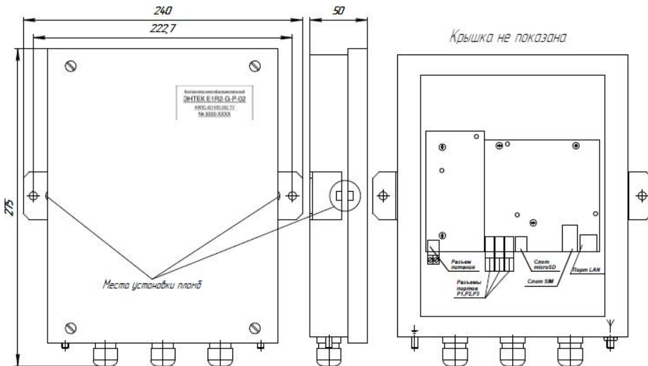
Рисунок 3. Места установки пломб КМ ЭНТЕК E1R2-G-P-02
