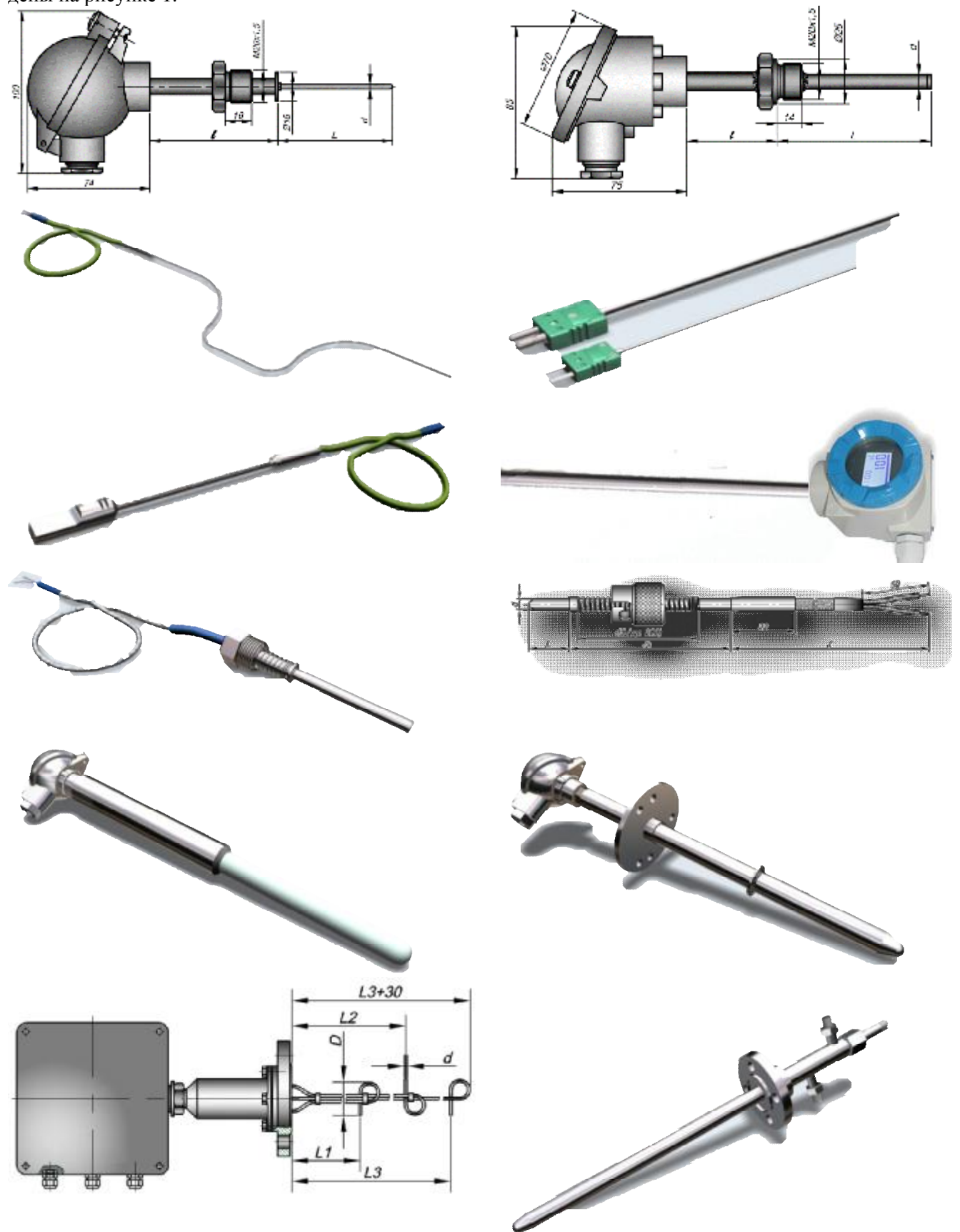
Рисунок 1 – Датчики температуры КТХА, КТНН, КТХК, КТЖК, КТМК
