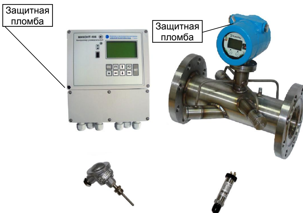
Рисунок 2 — Счётчик газа ультразвуковой СГУ.2
