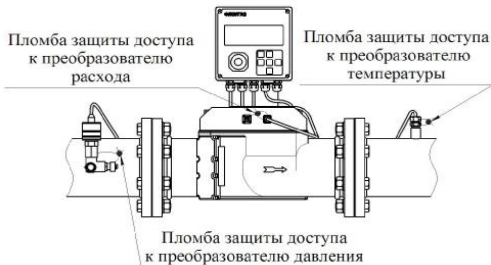
Рисунок 2 – Схема пломбирования комплекса
