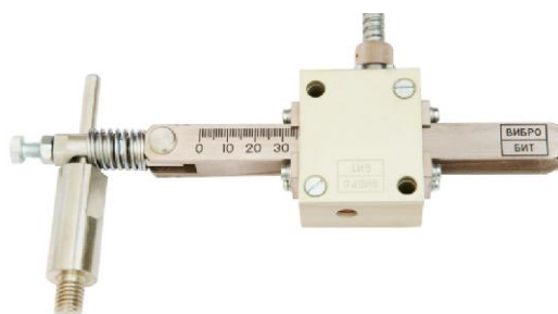
Рисунок 8 - Общий вид датчика вихретокового модификации RS400.050 со штоком
