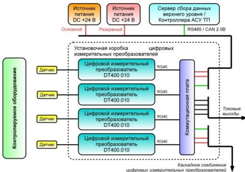
Рисунок 2 - Структурная схема
