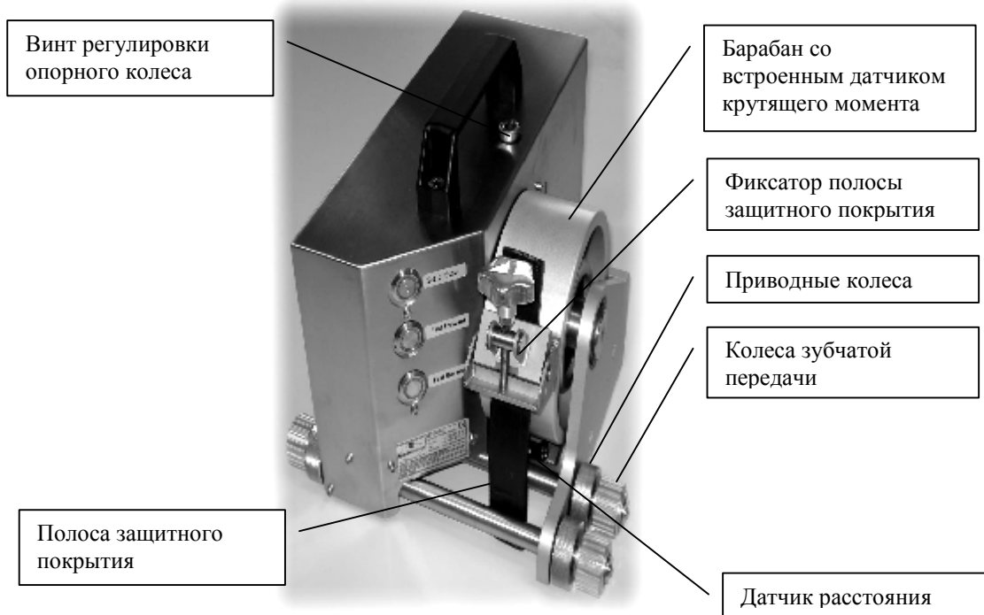
Внешний вид электромеханического блока адгезиметров электронных SPT 2500
