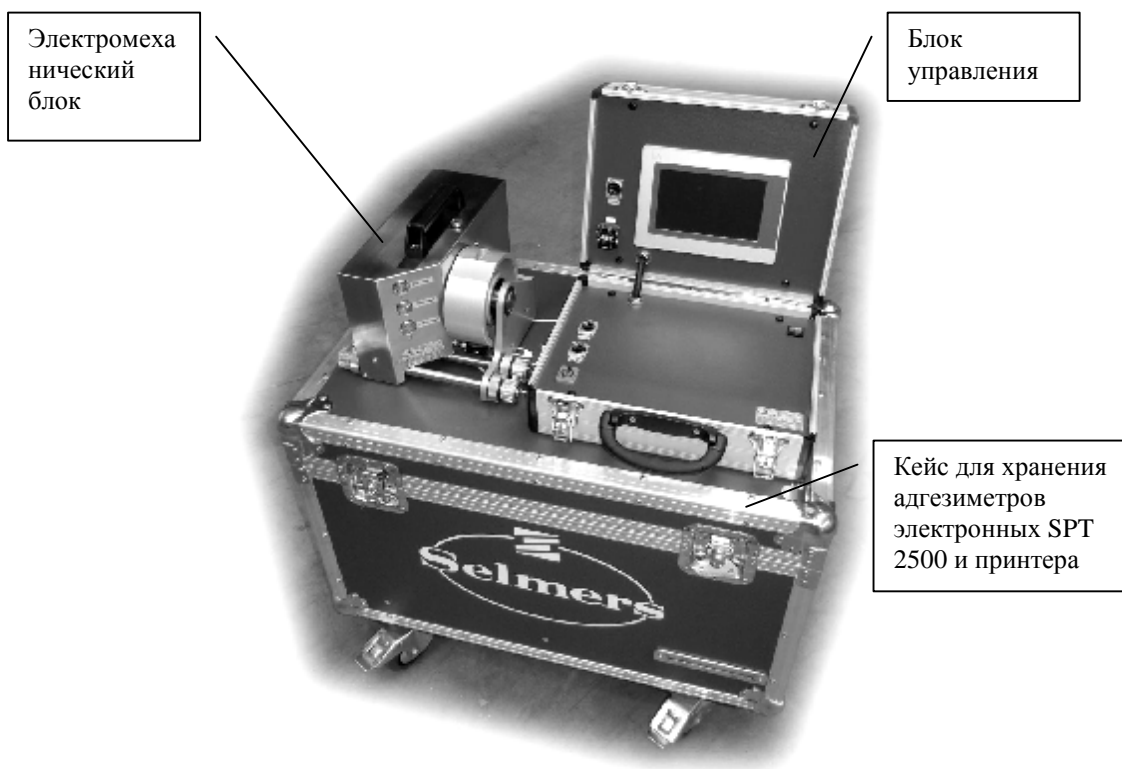
Общий вид адгезиметров электронных SPT 2500
