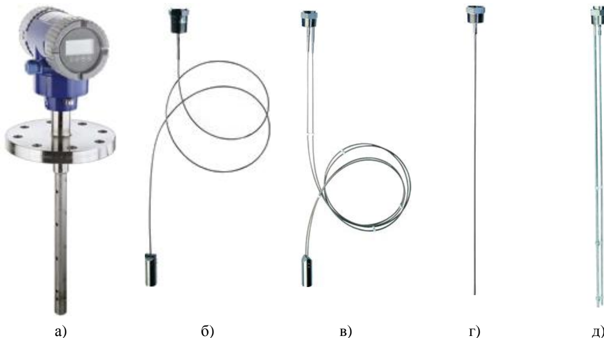
Р и с у н о к 1 – Уровнемеры LG01: а) общий вид уровнемера LG01 с коаксиальным волноводом, б) гибкий однопроводный волновод с грузом, в) гибкий двухпроводный волновод с грузом, г) жёсткий одностержневой волновод, д) жёсткий двухстержневой волновод.
