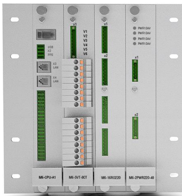
Рисунок 5 - Внешний вид контроллера на 4 слота (вид со стороны установки модулей, в зависимости от кода заказа внешний вид контроллера может изменяться). Место нанесения знака утверждения типа аналогично предыдущим вариантам
