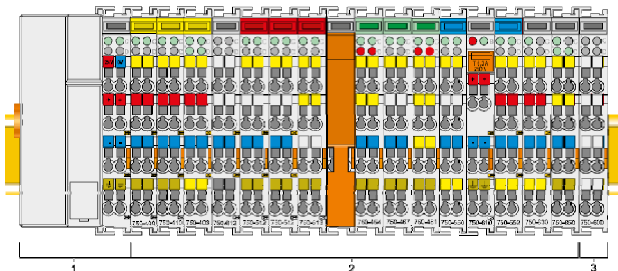
Рисунок 2 – Узел полевой шины
