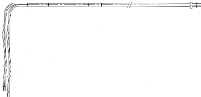
Рис. 1 Внешний вид преобразователя термоэлектрического с двумя термопарами модели 1133-11-733/3*5000.
