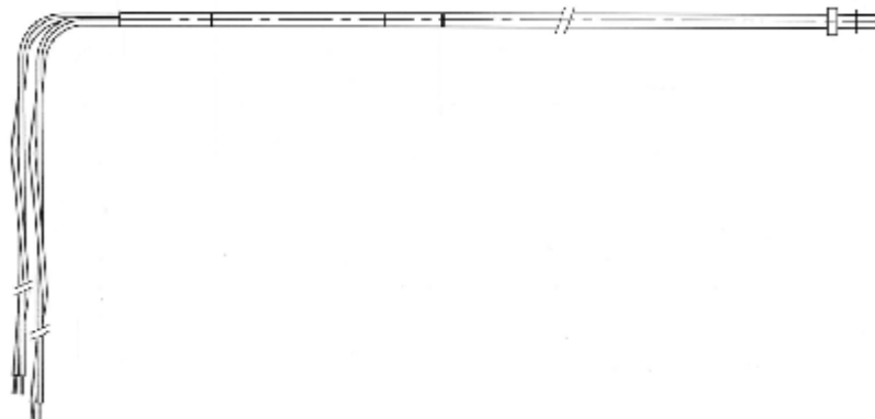
Рис. 1 Внешний вид преобразователя термоэлектрического с двумя термопарами модели 1133-11-2074/3*3000
