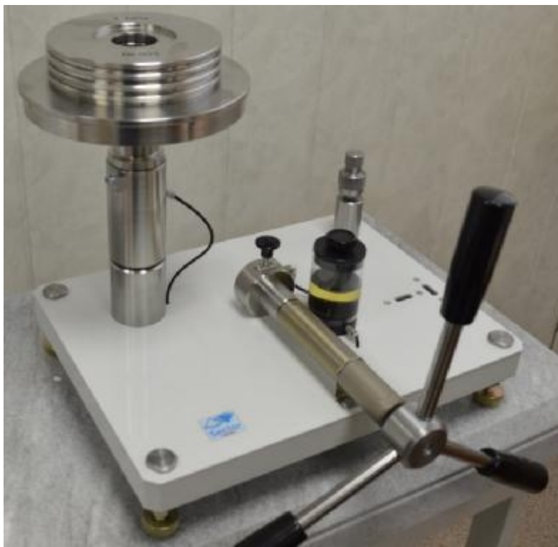
Рисунок 1 – Манометр грузопоршневой МП-600
