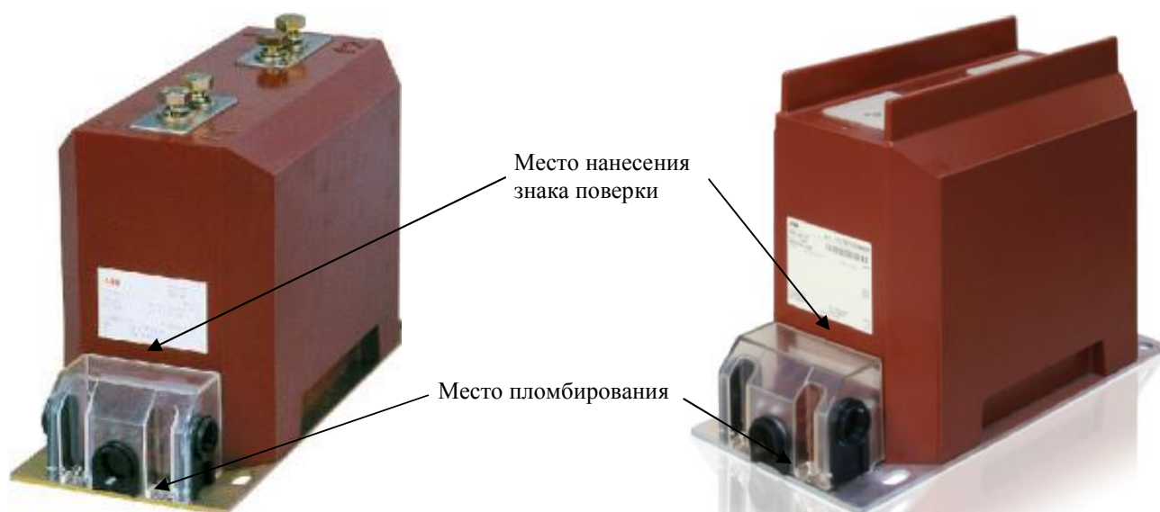
Рисунок 1 - Внешний вид трансформаторов тока TPU 4X.XX
