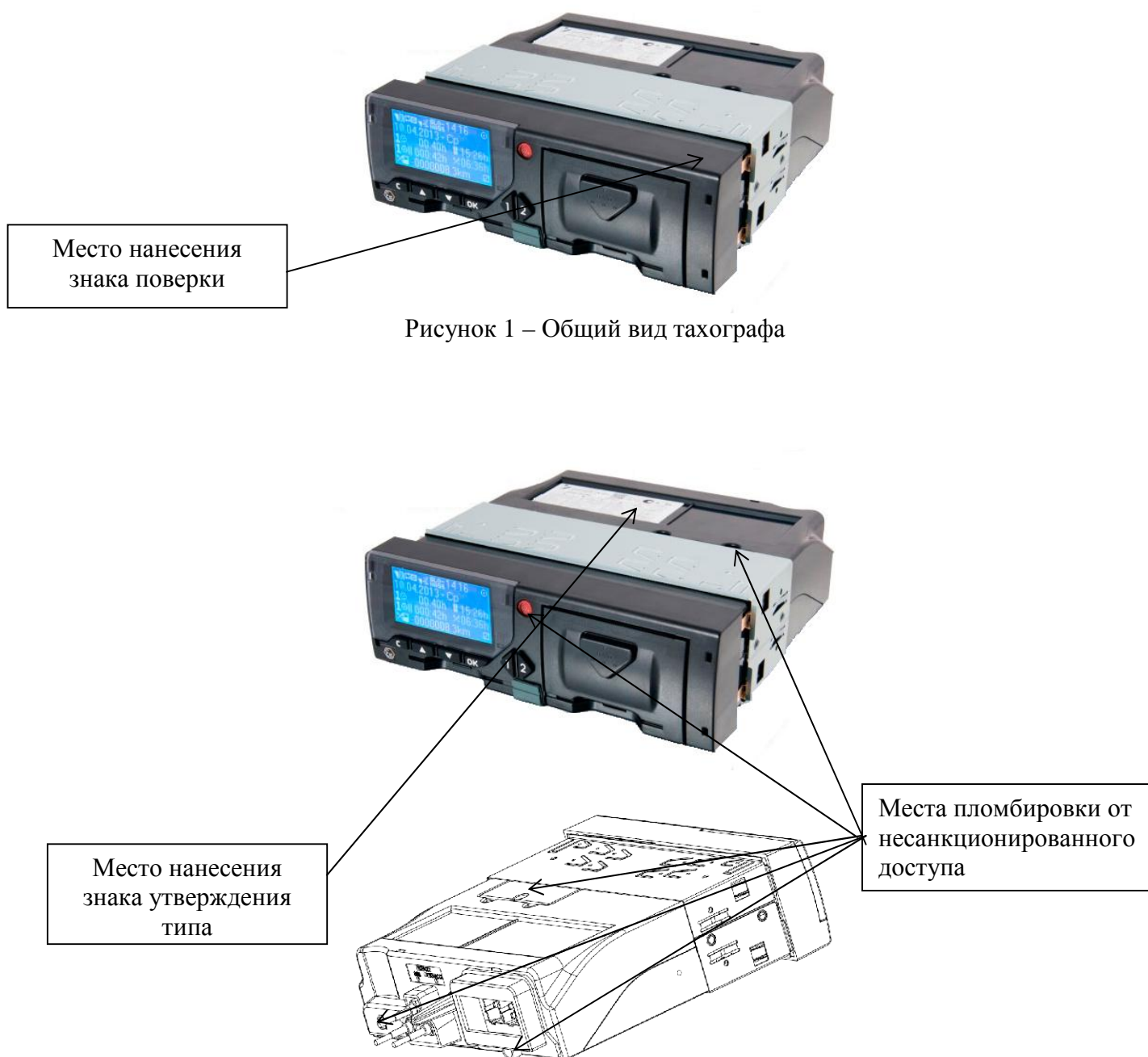
Рисунок 2 – Схема пломбировки от несанкционированного доступа и место нанесения знака об утверждении типа
