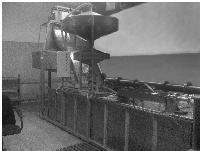
Рисунок 1 – Общий вид установки поверочной автоматизированной АКВА-200АМ
