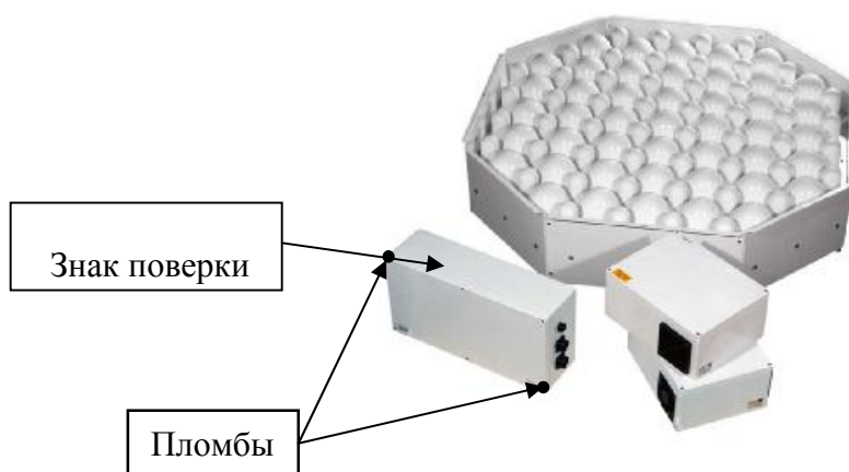
Рисунок 2 - Схема пломбирования и размещения знака поверки содаров FAS
