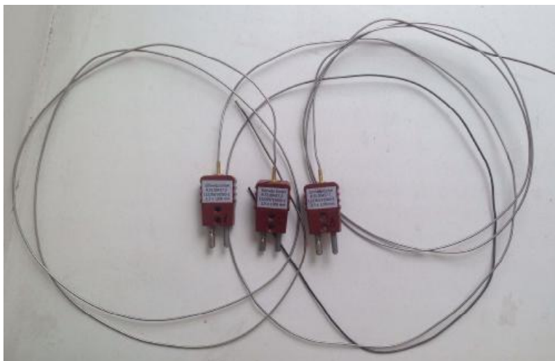
Рисунок 1 – Внешний вид преобразователей термоэлектрических 9.55.00457.3
