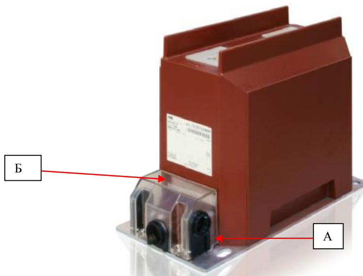
Рисунок 1 – Общий вид трансформатора тока ТРУ 40.23
