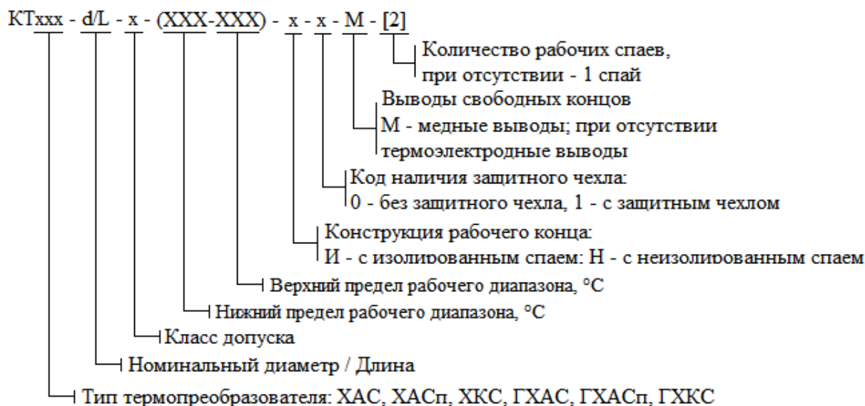
Рисунок 1 – Условное обозначение преобразователей термоэлектрических кабельных
