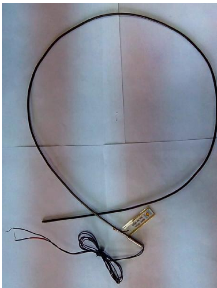
Рисунок 2 – Внешний вид преобразователей термоэлектрических кабельных КТХАС, КТХАСп и КТХКС
