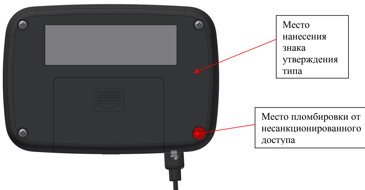
Рисунок 4 - Схема пломбировки от несанкционированного доступа и место нанесения знака об утверждении типа (исполнение корпуса 02)
