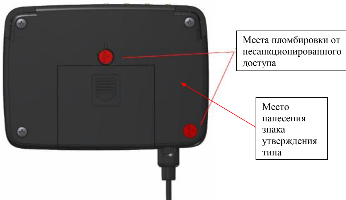
Рисунок 3 - Схема пломбировки от несанкционированного доступа и место нанесения знака об утверждении типа (исполнение корпуса 01)
