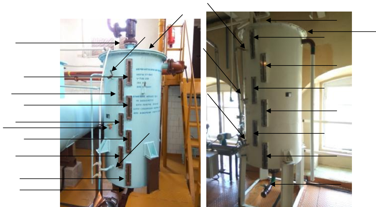
Рисунок 1 - Общий вид и места пломбирования мерника
