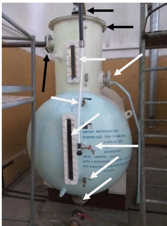
Рисунок 1 - Общий вид и места пломбирования мерника
