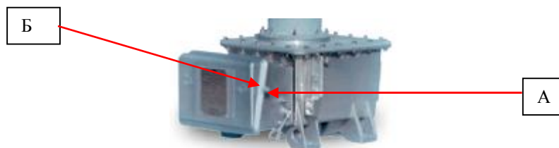
Рисунок 2 - Место пломбировки от несанкционированного доступа (А) и обозначение места нанесения знака поверки (Б)
